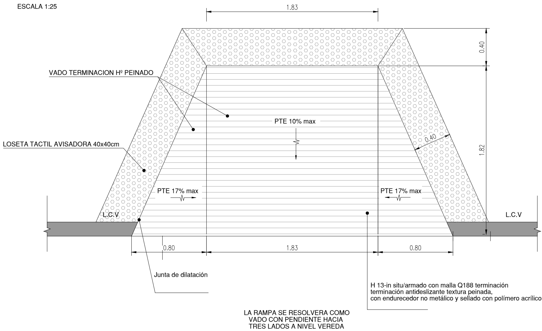
CORTE ESCALA 1:25
