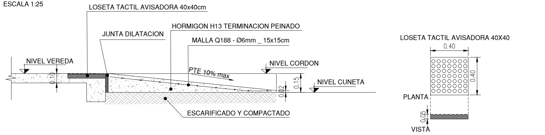
CORTE ESCALA 1:25
