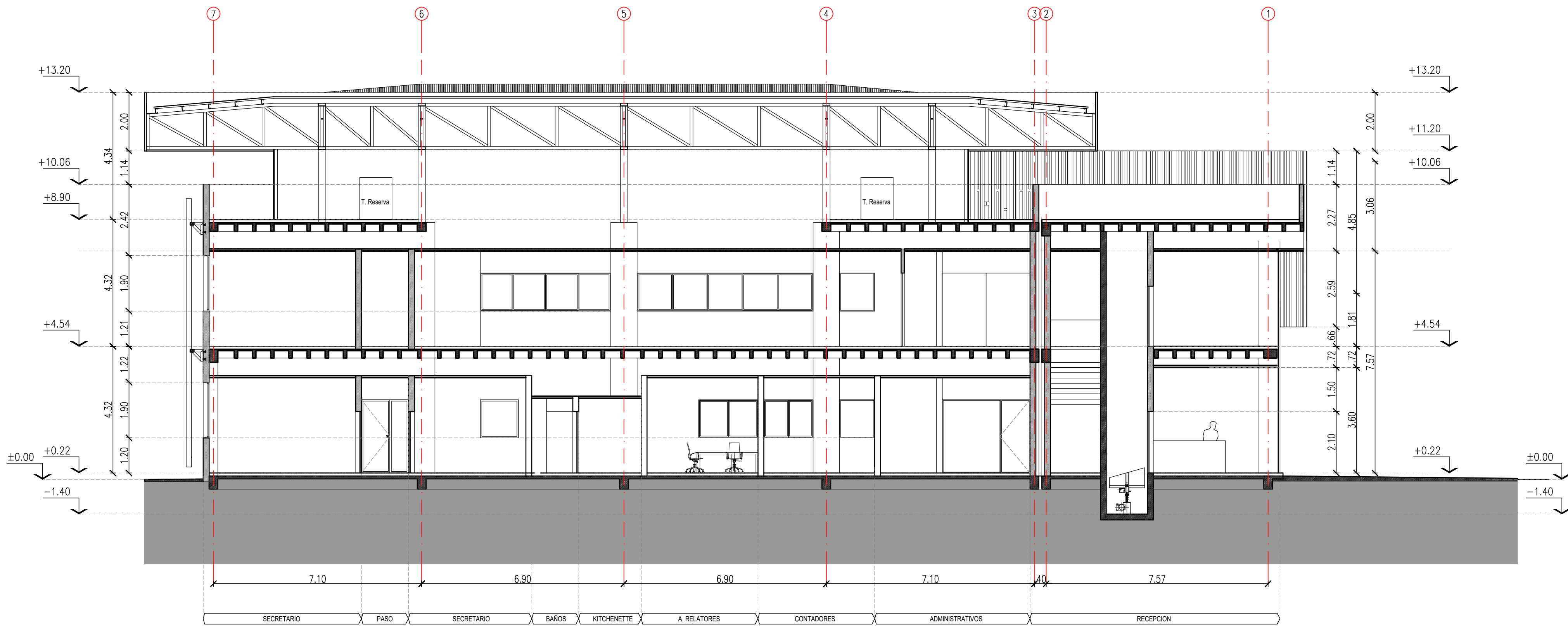
CORTE 1-1 ESC. 1:100
