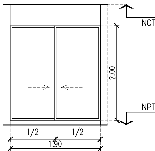
VISTA
