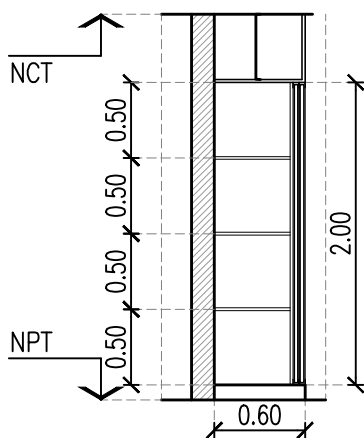
CORTE
