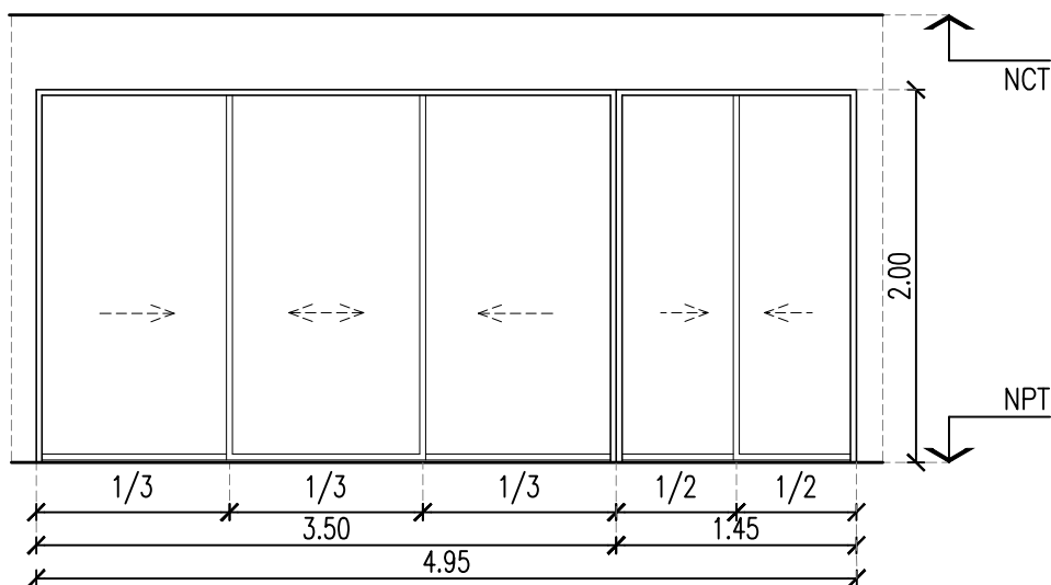
VISTA
