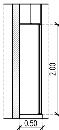
CORTE
