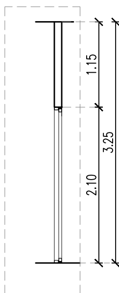
CORTE
