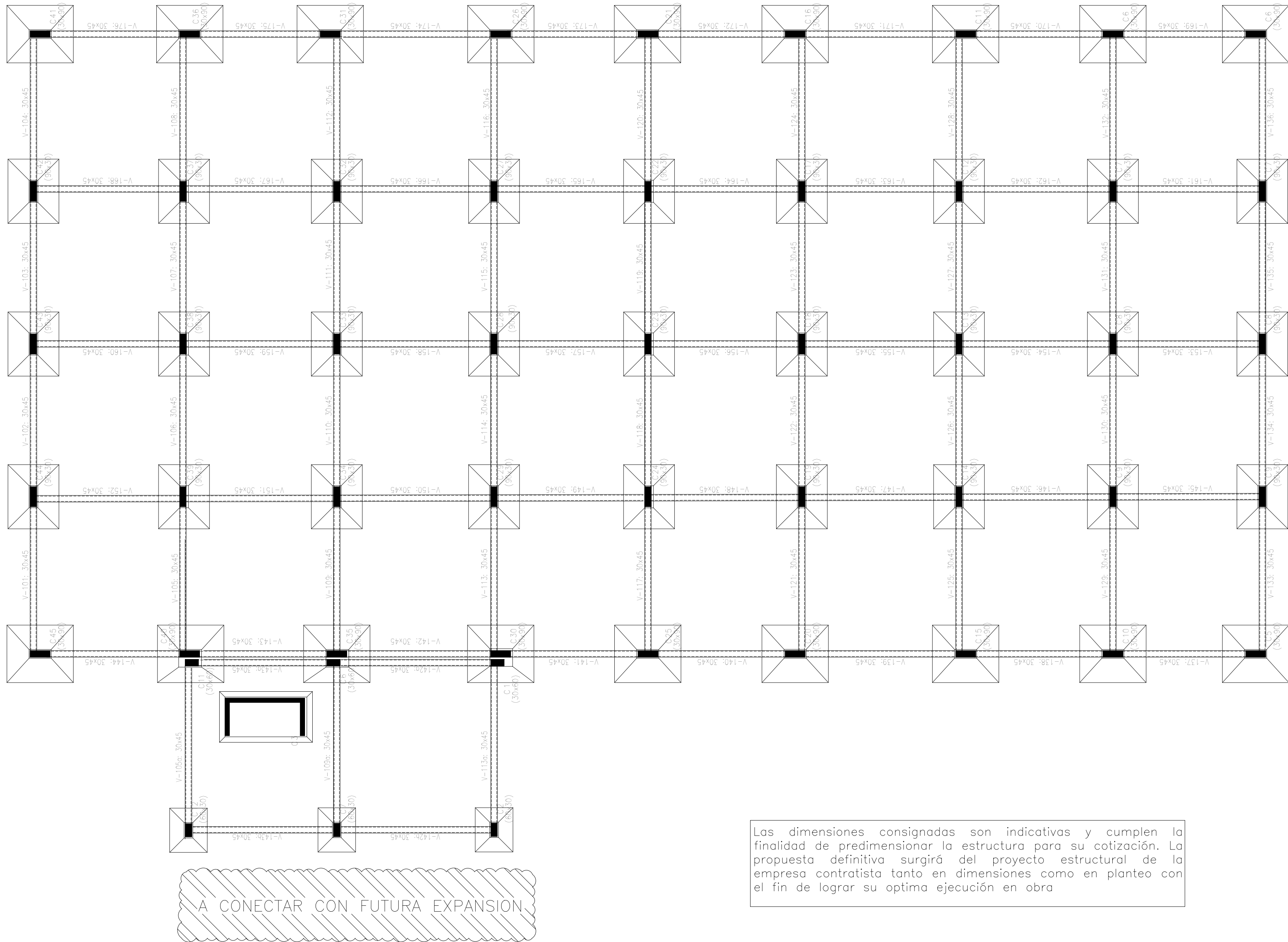
FUNDACIONES VIGA ENCADENADO INFERIOR
