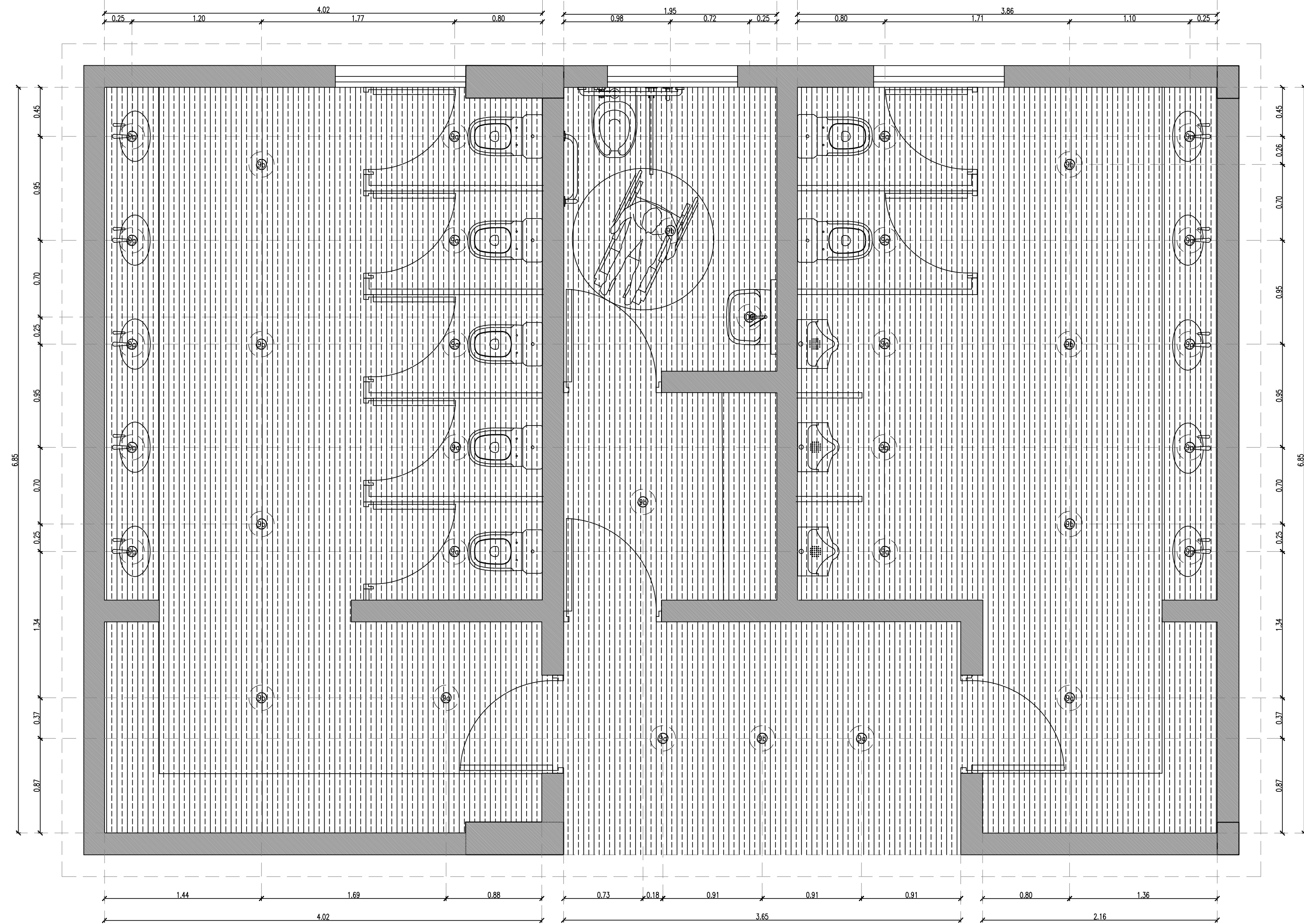
PLANTA CIELORRASO ESC.1:50
