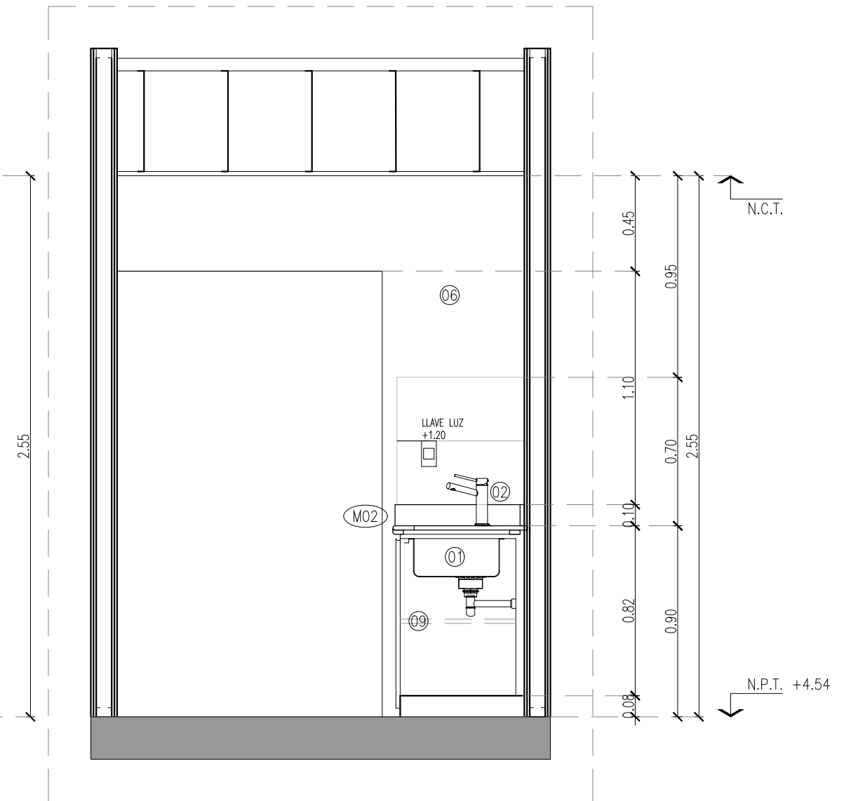
CORTE 1-1
