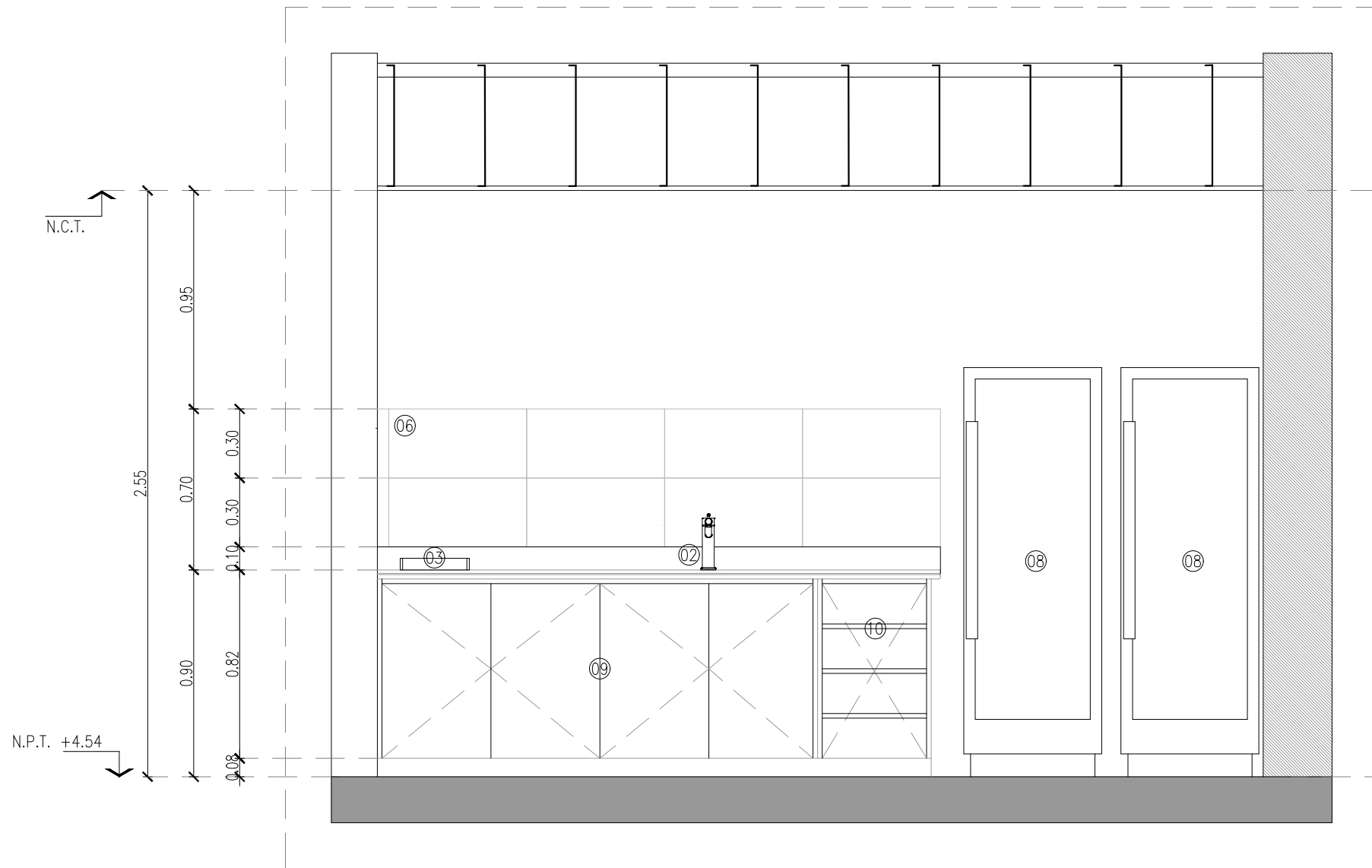
CORTE 2-2
