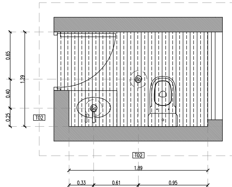
PLANTA CIELORRASO ESC.1:20
