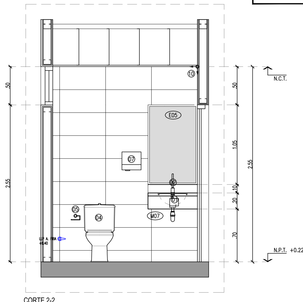
CORTE 2-2
