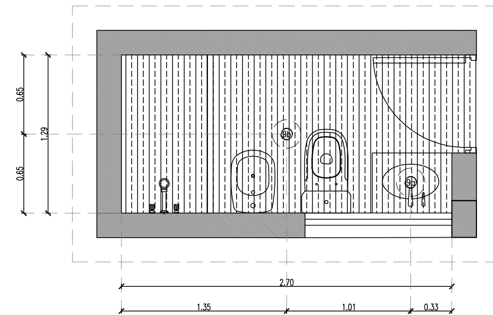
PLANTA CIELORRASO ESC.1:20
