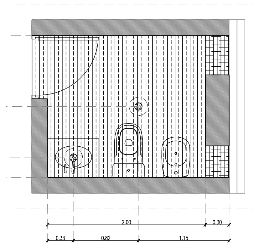
PLANTA CIELORRASO ESC: 1:20
