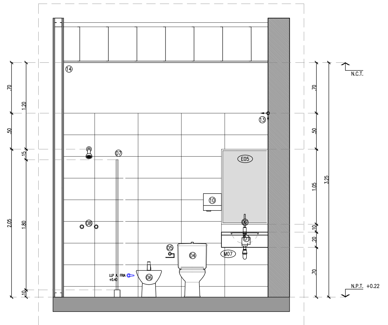
CORTE 2-2
