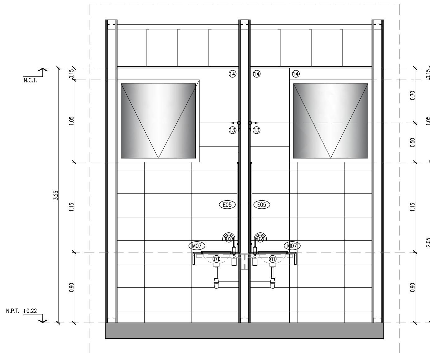
CORTE 1-1
