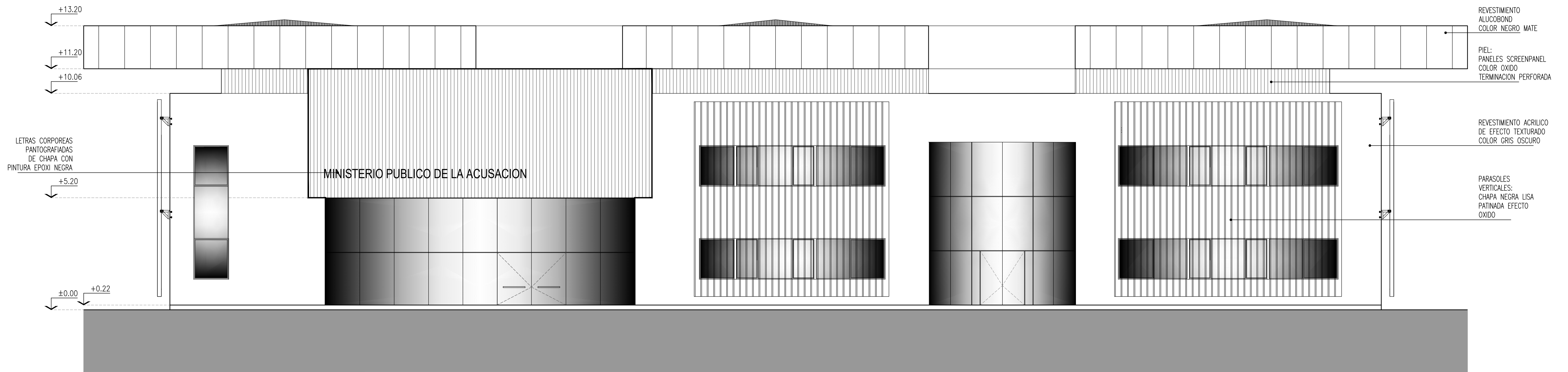
ELEVACION LATERAL IZQUIERDA ESC.1:100
