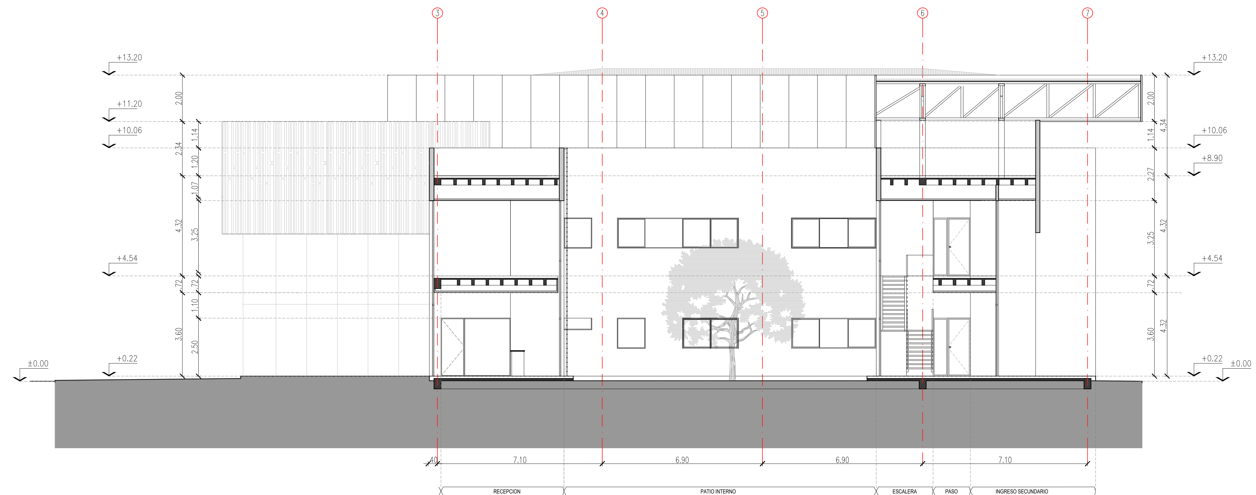
CORTE 3-3 ESC. 1:100
