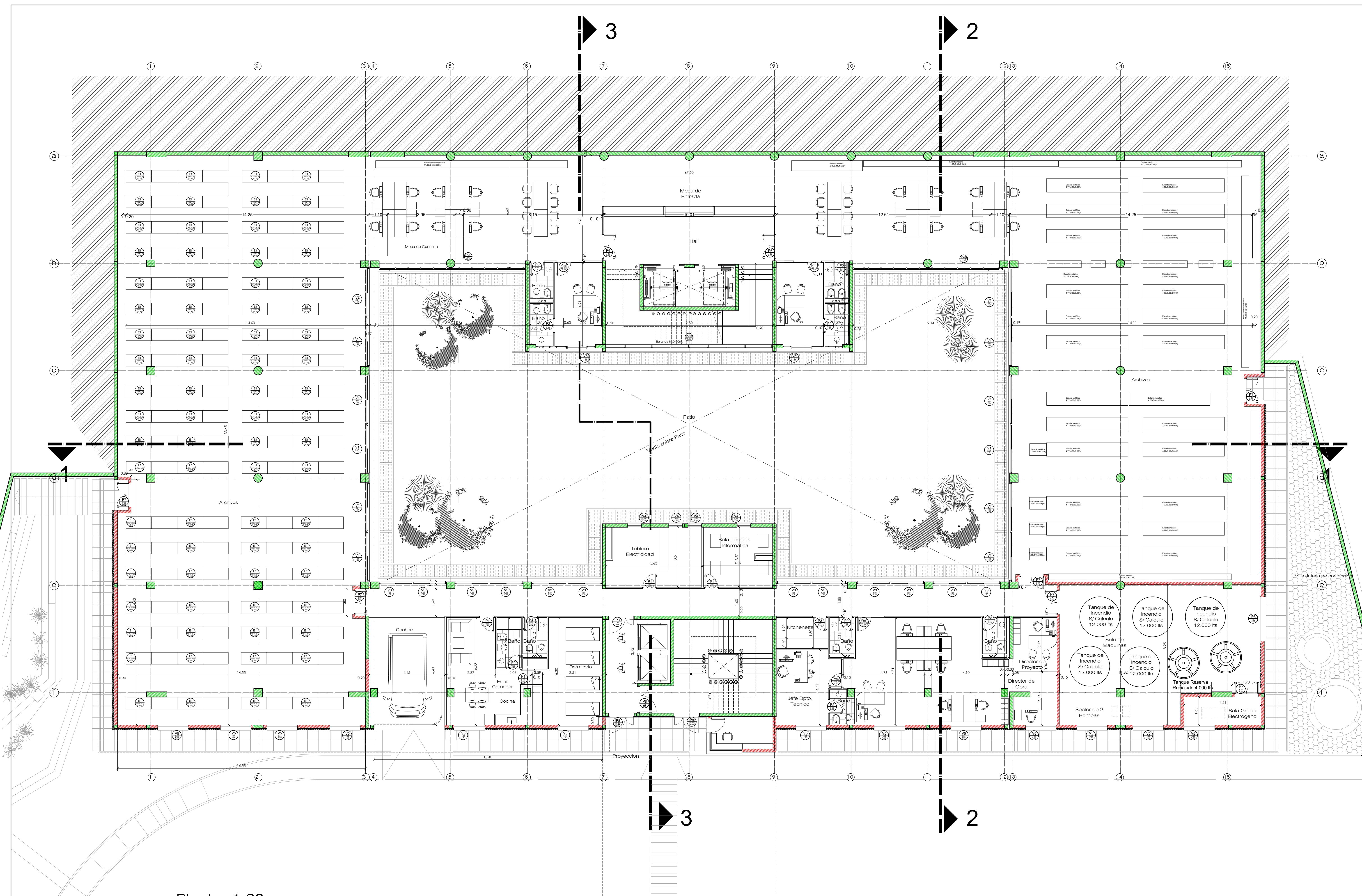
Planta -1.80
