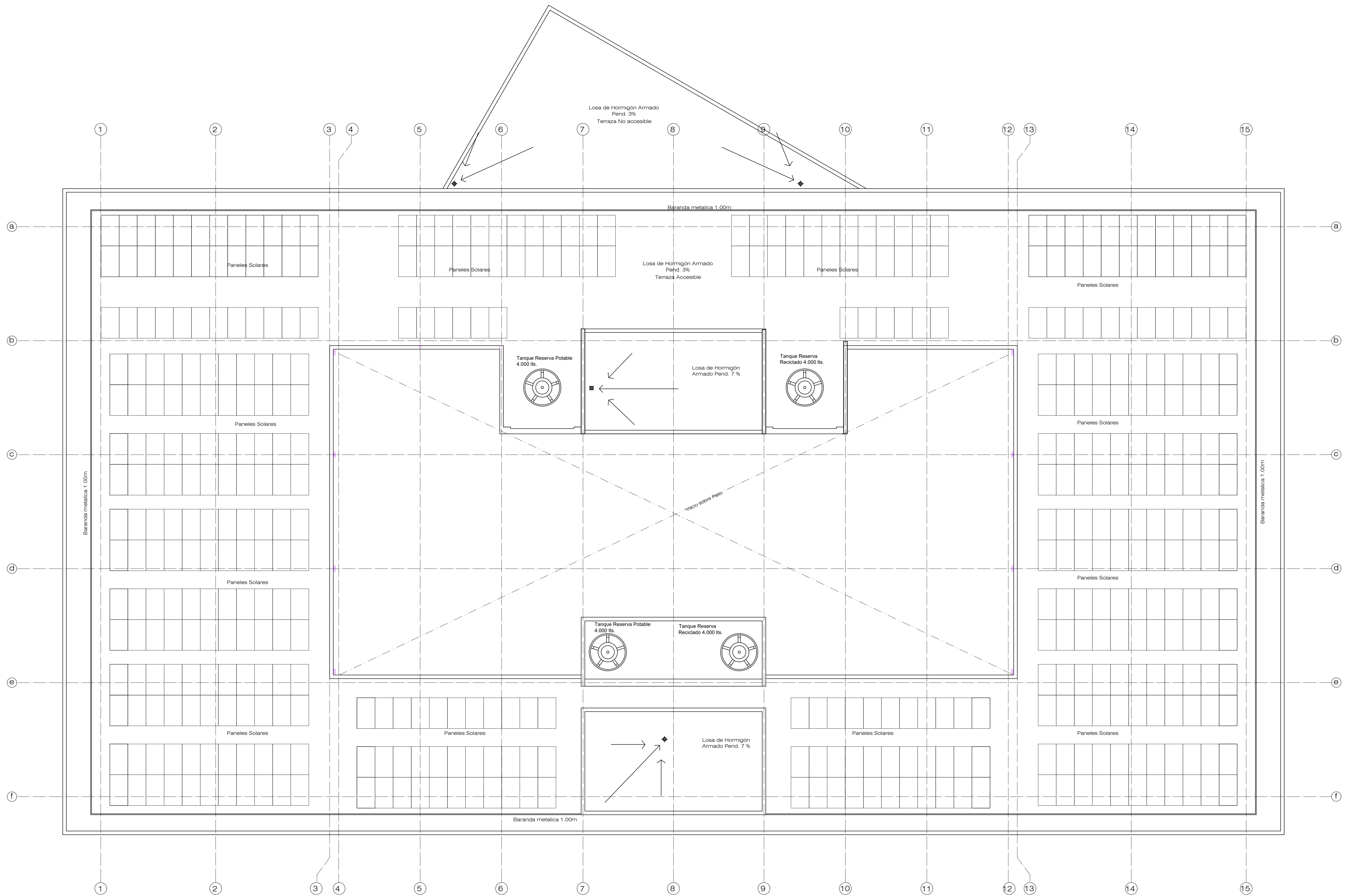
Planta de Techos +25.28
