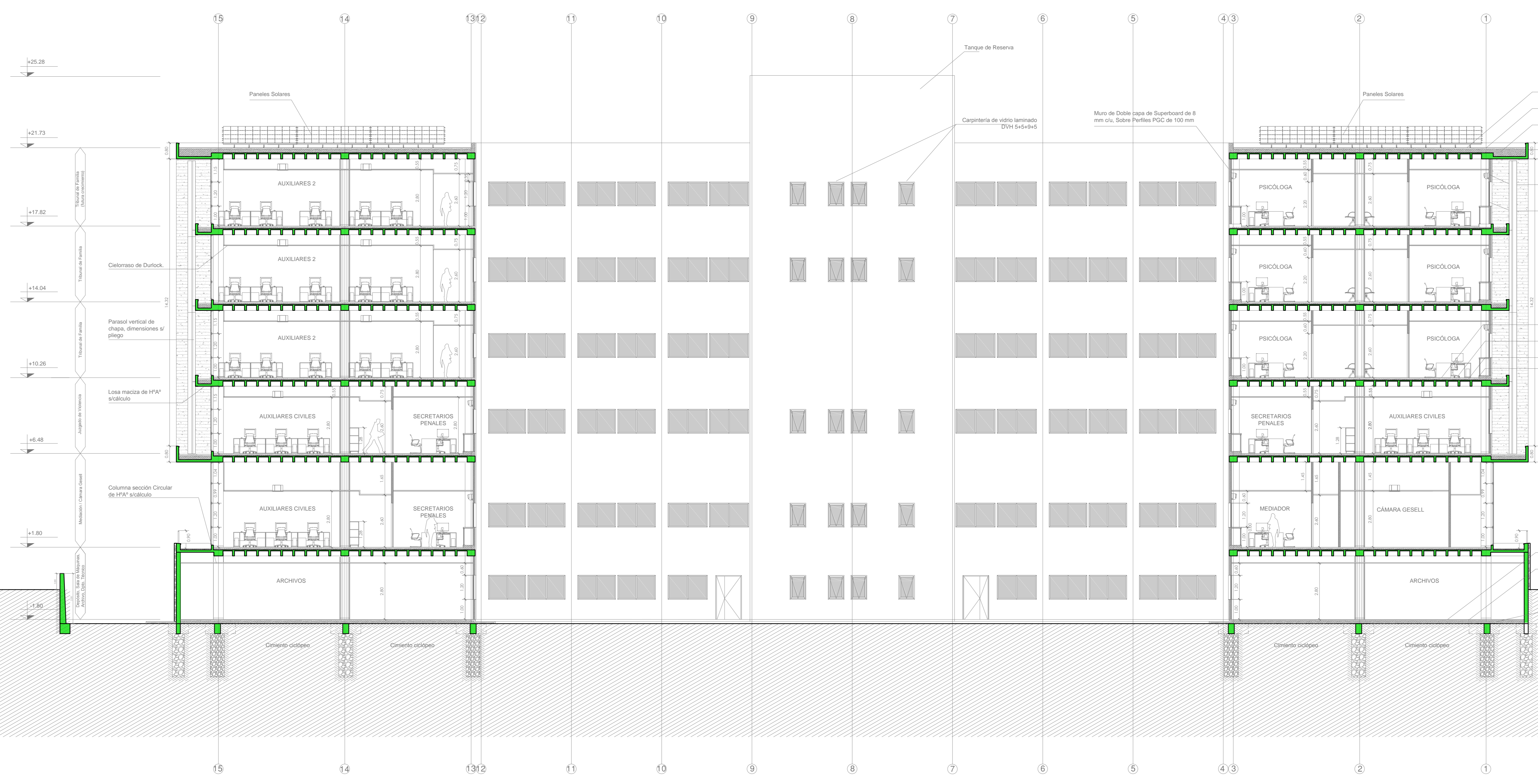
CORTE LONGITUDINAL 1-1
