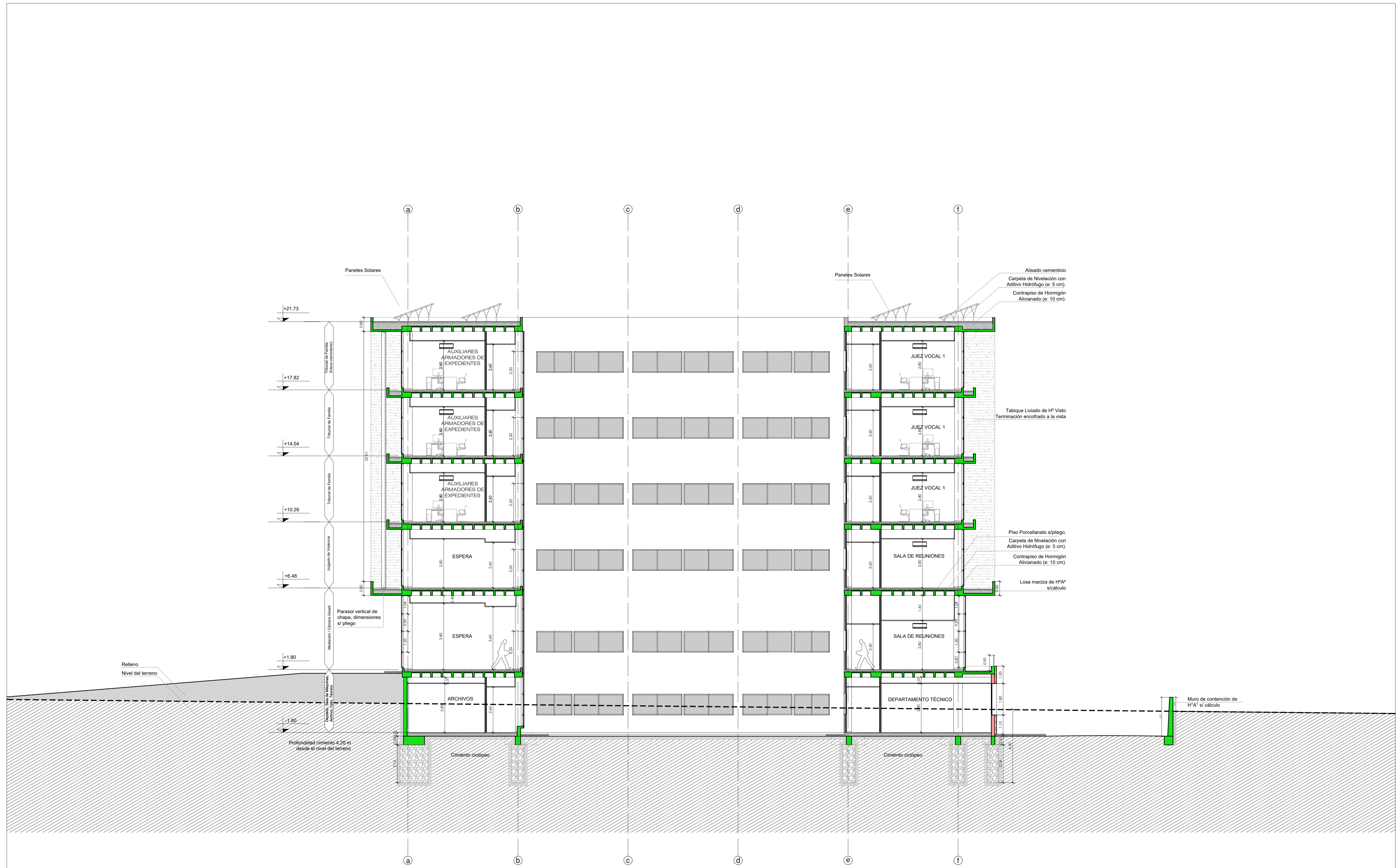
CORTE TRANSVERSAL 2-2
