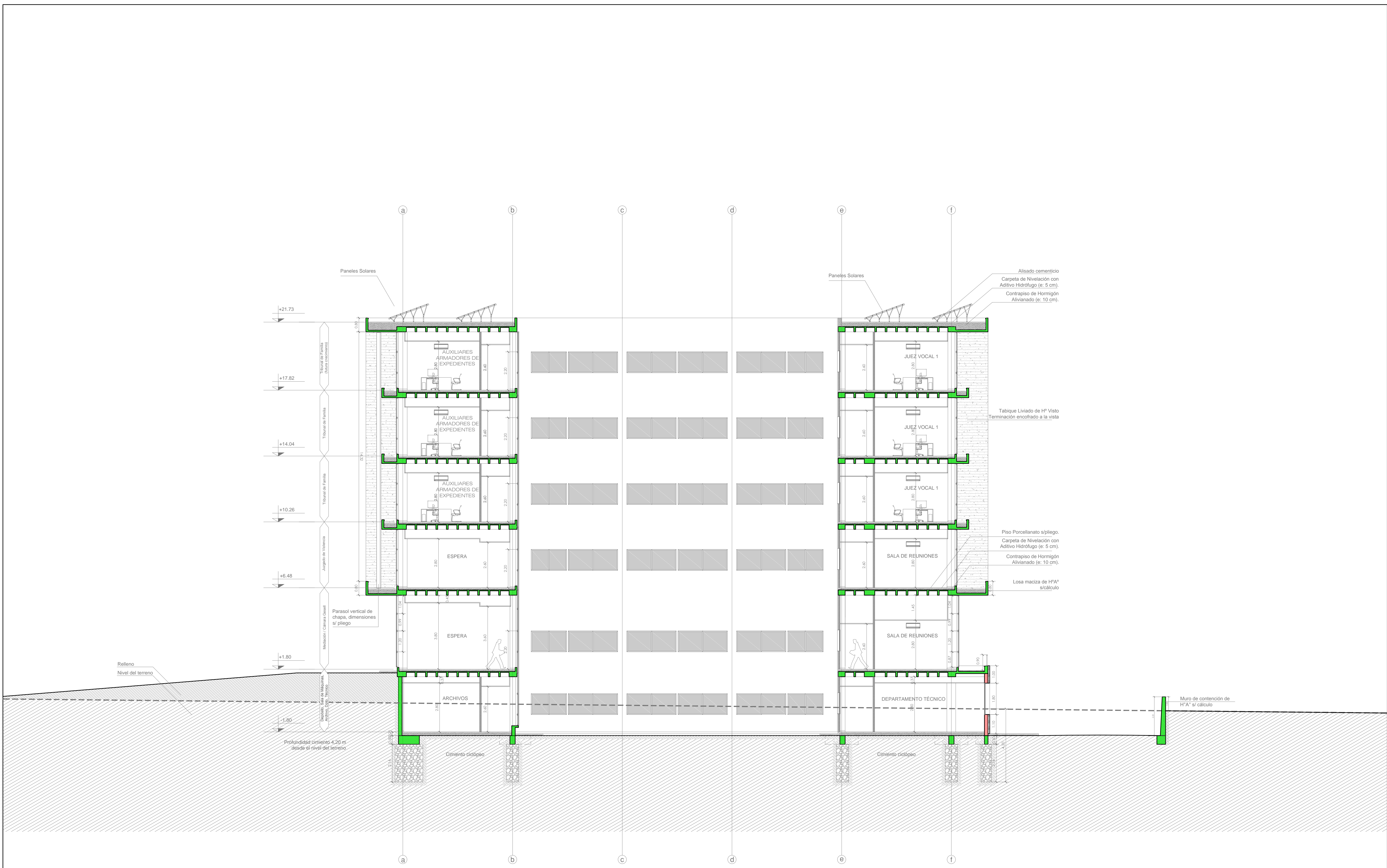
CORTE TRANSVERSAL 2-2
