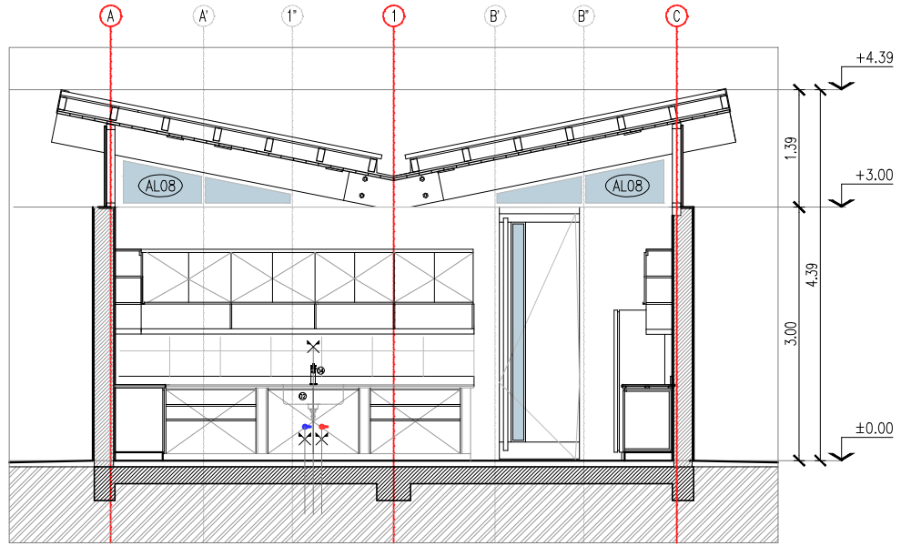
CORTE 1-1 ESC. 1:20
