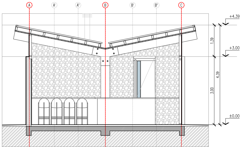
CORTE 2-2 ESC. 1:20
