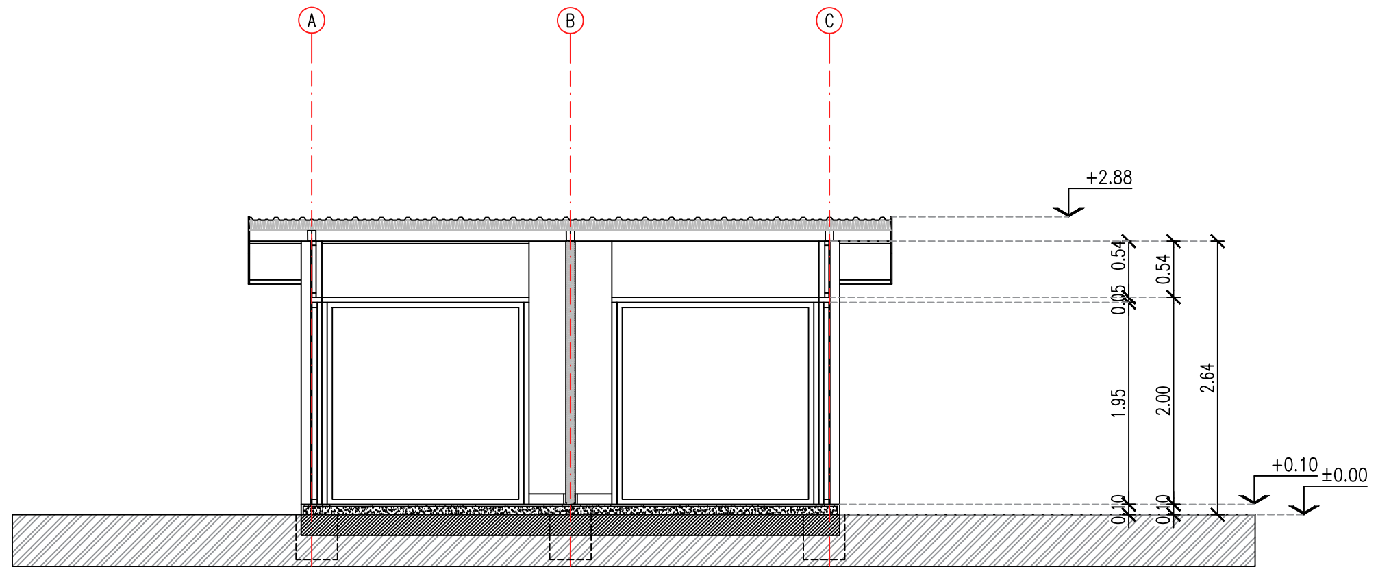
CORTE A-A
