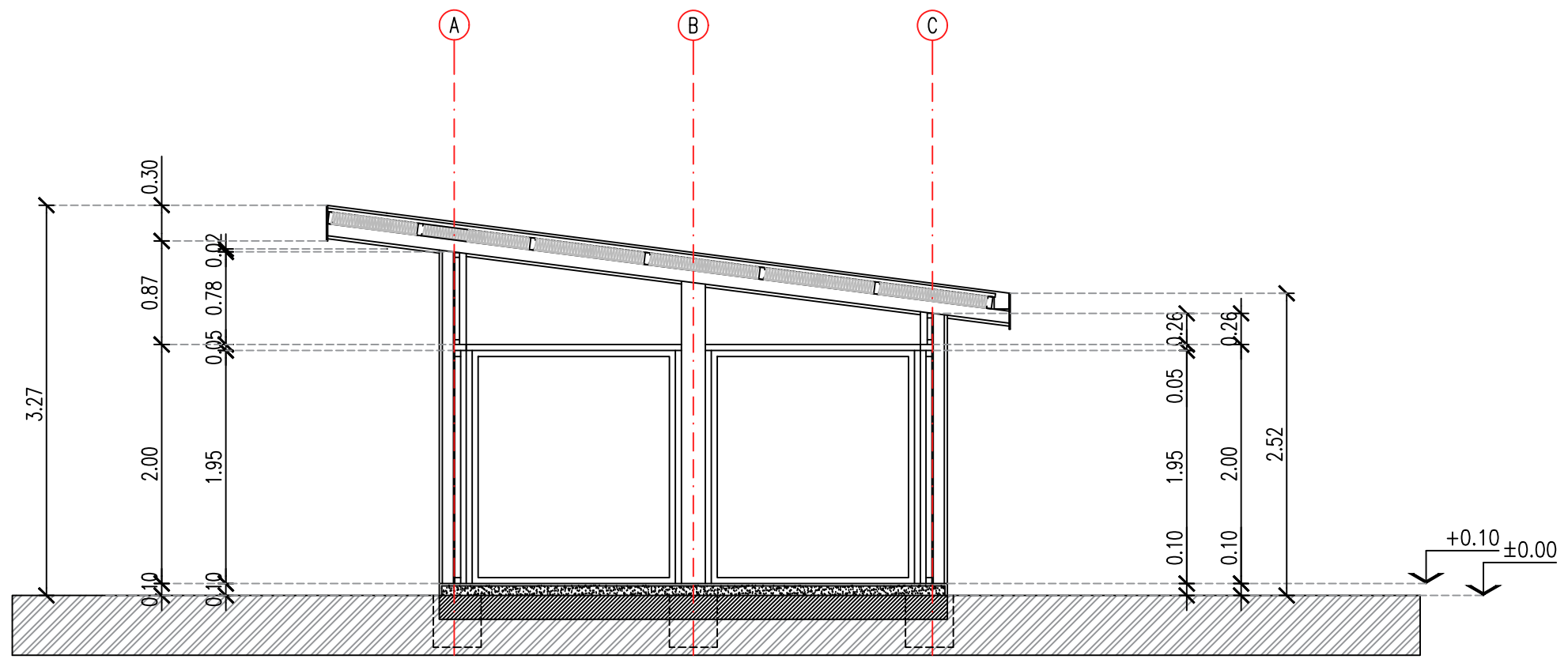
CORTE B-B
