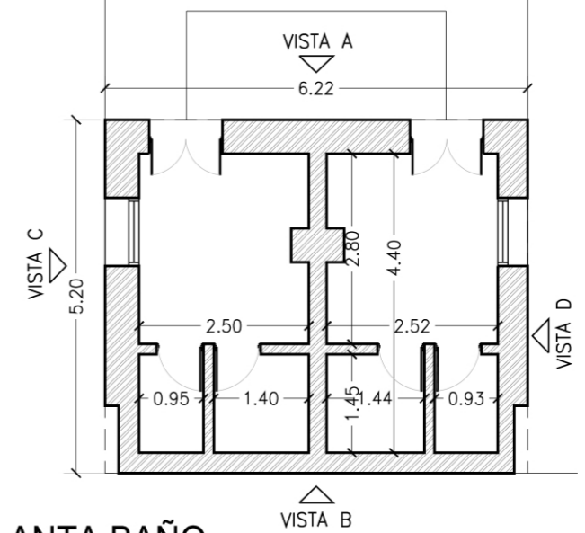
PLANTA BAÑO 1:100
